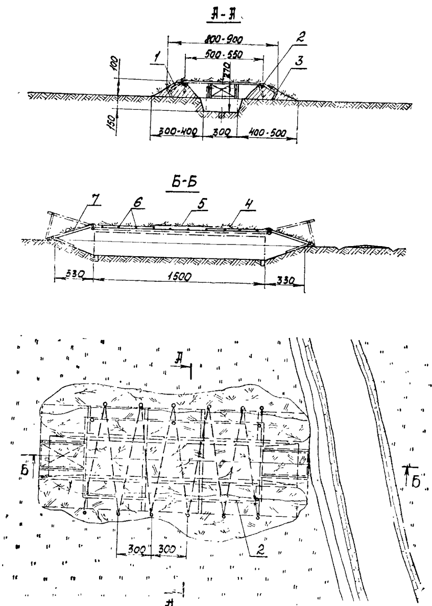
Рис. 137. Устройство маски-перекрытия над укрытием для имущества: 1 — засыпка грунтом; 2 — жерди (опоры для тяжёлых); 3 — анкерный кол; 4 — срезанная растительность или другой местный маскировочный материал; 5 — брезент или маскировочное покрытие; 6 — тяжёлый из гроя, проволоки или пенькового каната; 7 — откидная рама
