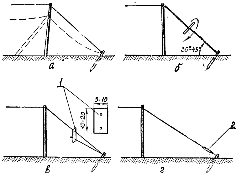
Рис. 33. Способы подтягивания тросов:
