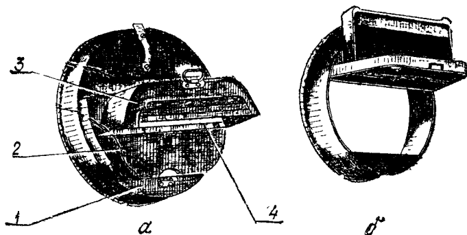
Рис. 46. Светомаскировочная насадка для фар:
