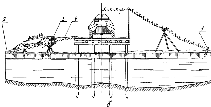
Рис. 130. Скрытие моста на замерзшей реке:
