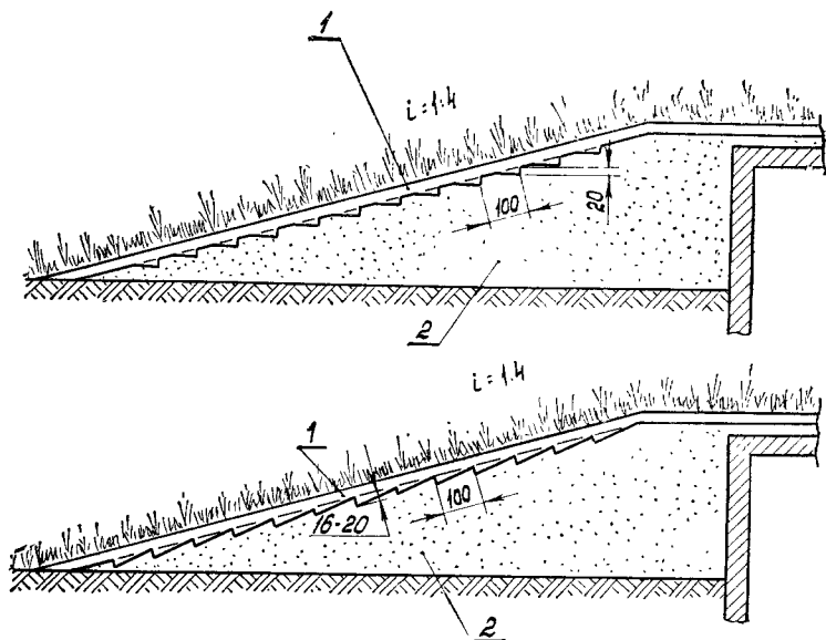
Рис. 58. Закрепление растительного слоя на обвалаваниях:
