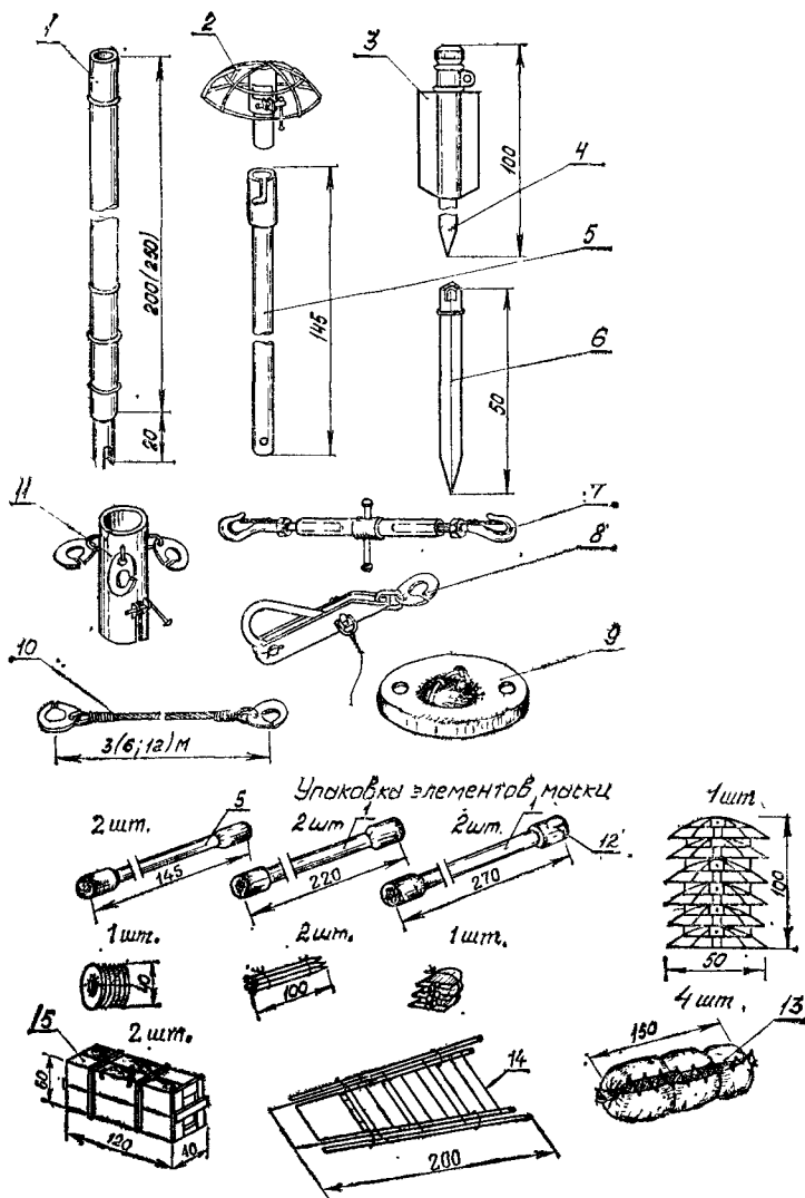
Рис. 20. Элементы универсальной каркасной маски УМК:
