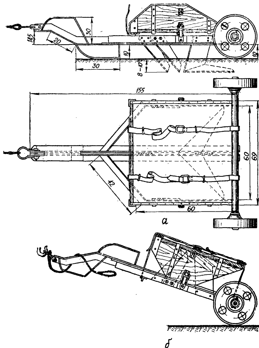
Рис. 57. Дернорез:
