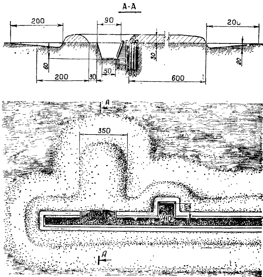
Рис. 121. Ложный участок траншей с ложным блиндажом и ложной ячейкой для стрелка
