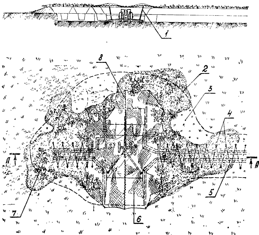
Рис. 117. Маскировка окопа для гаубицы:
