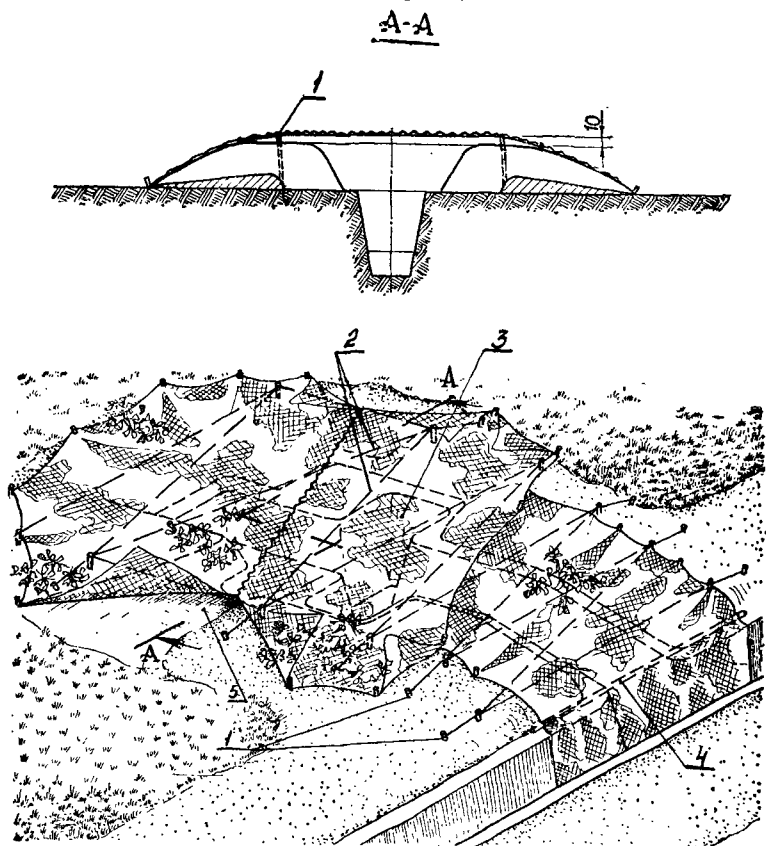
Рис. 106. Маскировка вынесенной площадки для пулемета:
