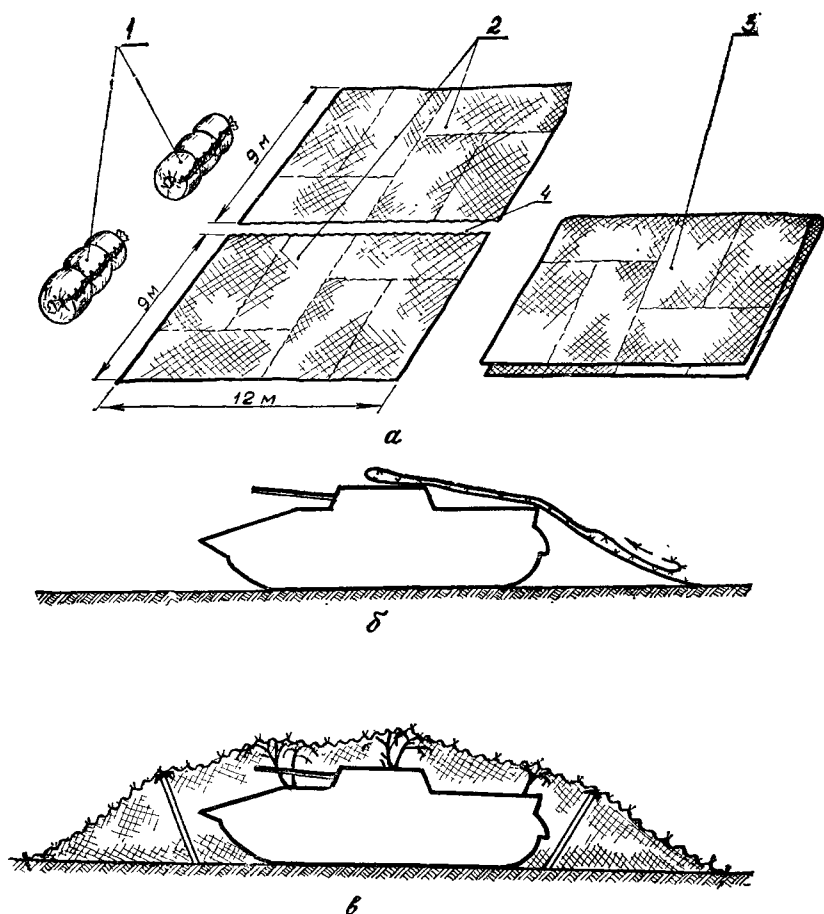
Рис. 100. Порядок установки маски-перекрытия из комплекта МКС-2М: а — развертывание и подготовка маскировочного покрытия; б — укладка покрытия на маскируемую технику; в — придание маске формы, отличающейся от формы техники; 1 — упаковка маскировочного комплекта; 2 — развернутые покрытия, 3 — складывание покрытий в два слоя; 4 — место сшивного шва
