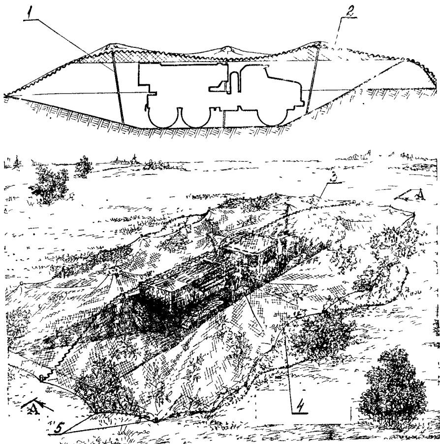
Рис. 118. Маскировка окопа для боевой машины реактивной артиллерии: 1 — стойка-подпорка; 2 — маскировочное покрытие, 3 — быстро распускающийся шов; 4 — наброска травы и реток, 5 — козья диаметром 6 см На маскировку требуется 8 чел.-ч. табельных масок «Шатер» — 1 шт.; местного мас- кировочного материала — 1 м 3
