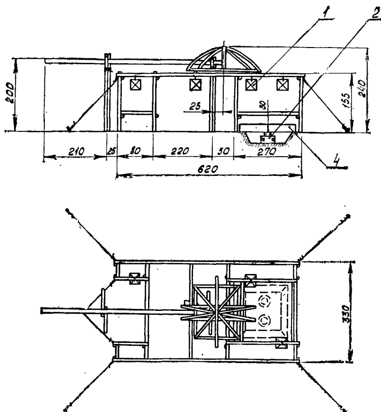
Рис. 66. Макет замаскиро
