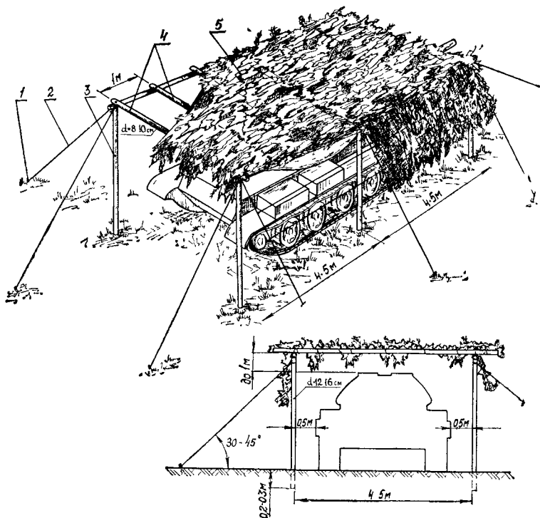
Рис. 36. Маска-навес:
