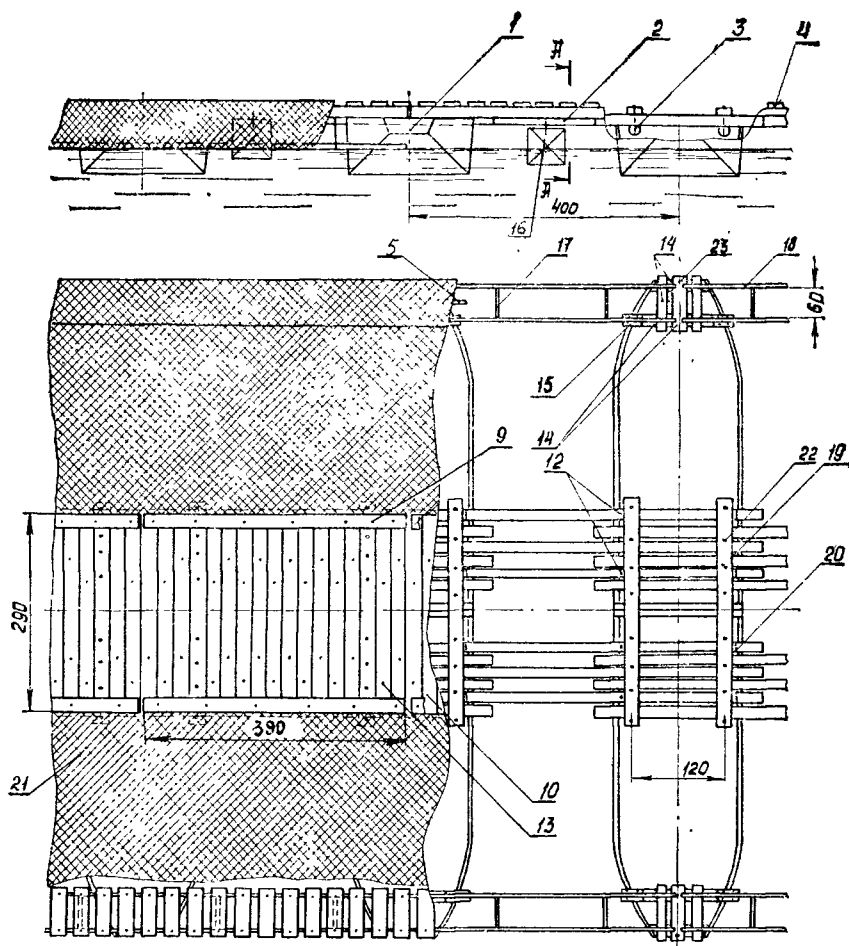
Рис. 133. Ложный наплавной мост на лодках ДЛ-10 для имитации моста ПМУП с давлением
