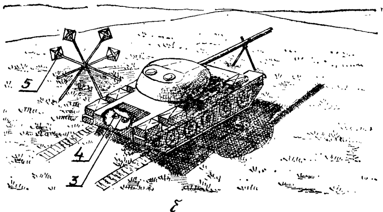
Рис. 81. Тепловой имитатор промышленного изготовления и его применение в макете танка:
