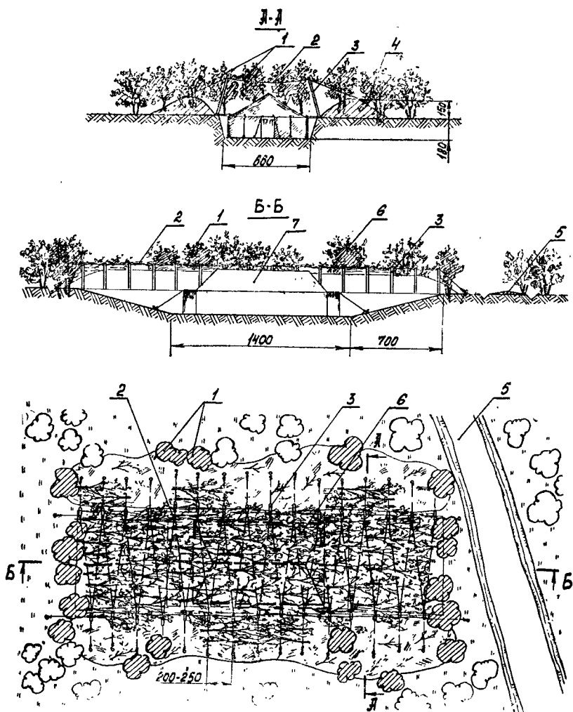
Рис. 141. Скрытие палатки, расположенной в укрытии:
