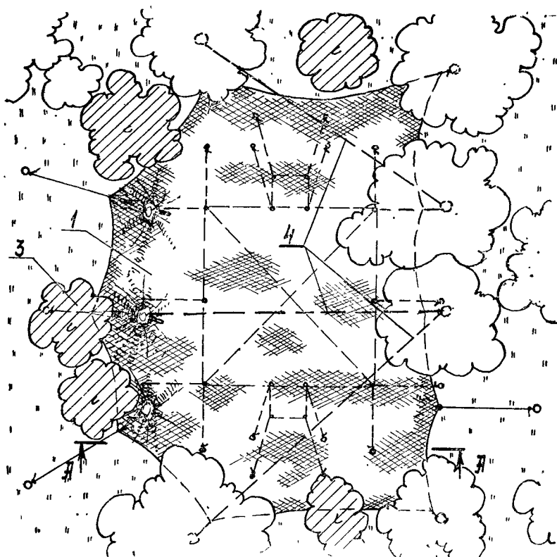
Рис. 140. Скрытые палатки табельным маскировочным комплектом:
