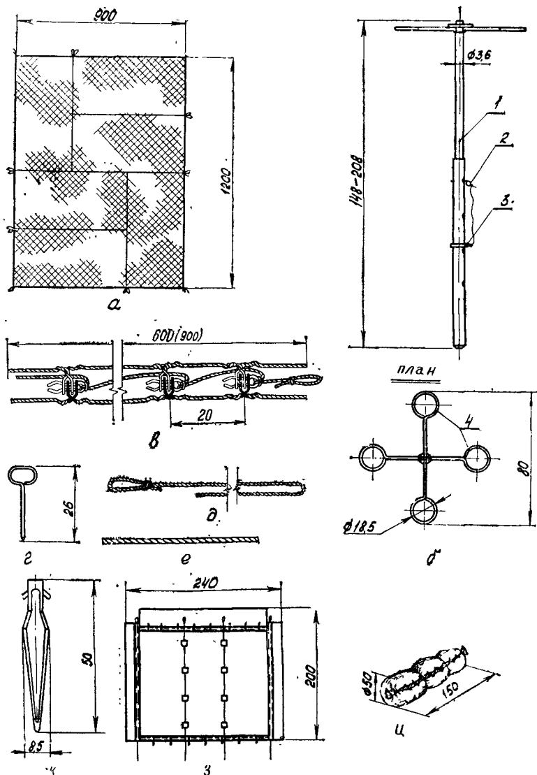
Рис. 16. Элементы табельного маскировочного комплекта МКС-2П:
