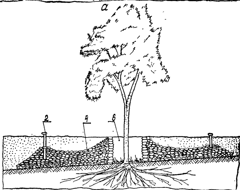
Рис. 64. Защита деревьев а — поперечный разрез законченного сухого колодца; б — поперечный разрез насыпи, соо насыпи; 1 — дренажная труба; 2 — вертикальная труба; 3 — рыхлая земля; 4 — наброска
