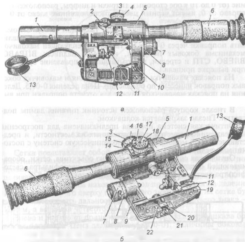
Рис. 81. Снайперский оптический прицел:
