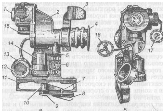
Рис. 88. Оптический прицел РПГ-7:
