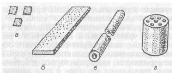
Рис. 48. Форма зерен бездымного пороха: а — пластинки; б — лента; в — трубка; г — цилиндр с семью каналами
