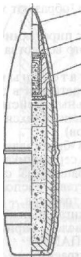
Рис. 118. Зажигательная пуля мгновенного действия МДЗ: 1 — наконечник; 2 — трубка рубящая; 3 — втулка с капсюлем-детонатором; 4 — прокладка; 5 — оболочка; 6 — стакан с взрывчатым веществом; 7 — рубашка
