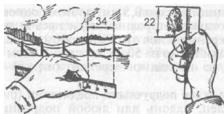
Рис. 154. Измерение вертикального и горизонтального углов с помощью линейки
