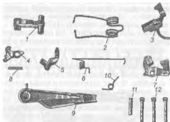
Рис. 64. Ударно-спусковой механизм:
