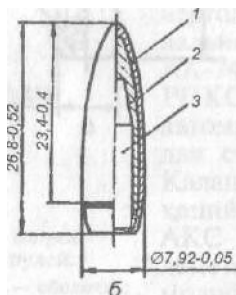
Рис. 134. 7,62-мм патрон образца 1943 г. с пулей со стальным сердечником: а — патрон; б — пуля; 1 — оболочка; 2 — сердечник свинцовый; 3 — сердечник стальной
