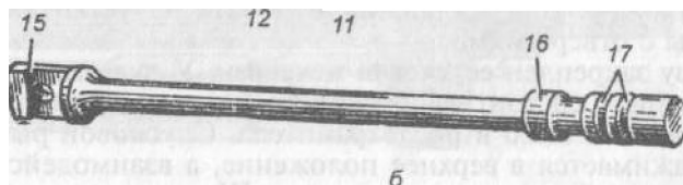
Рис. 76. Затворная рама с газовым поршнем:
