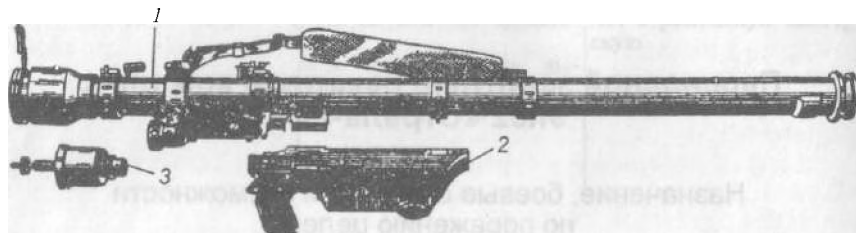
Рис. 107. Переносной зенитный ракетный комплекс 9К32: 1 — труба с ракетой 9М32; 2 — источник питания, отсоединенный от трубы; 3 — пусковой механизм
