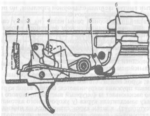
Рис. 72. Положение частей ударно-спускового механизма перед выстрелом:
