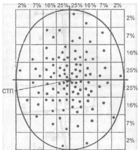
Рис. 22. Закономерность рассеивания
