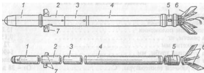
Рис. 108. Зенитная ракета 9М32: 1 — головной отсек; 2 — рулевой отсек; 3 — боевой отсек; 4 — двигательный отсек; 5 — хвостовая часть; 6 — крылья; 7 — рули
