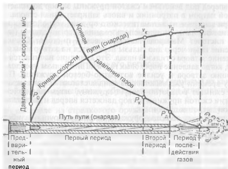
Рис. 1. Периоды выстрела:
