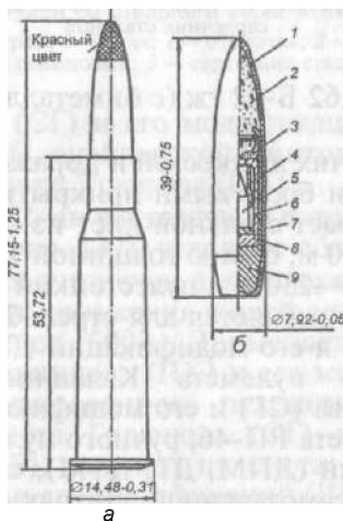
Рис. 139. 7,62-мм винтовочный патрон с пристрелочно-зажигательной пулей ПЗ:
