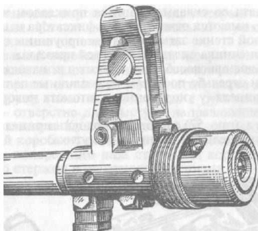
Рис. 55. Основание мушки
