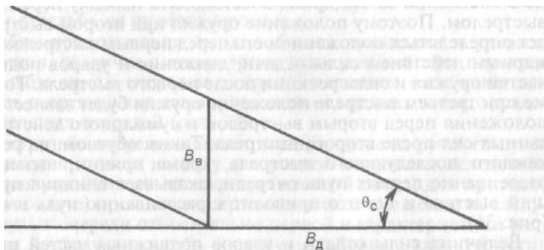
Рис. 30. Зависимость между срединными отклонениями по дальности ( B_d ) и по высоте ( B_v )
