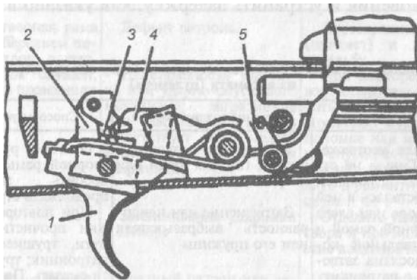
Рис. 73. Положение частей ударно-спускового механизма после одиночного выстрела: / — спусковой крючок; 2 — замедлитель курка; 3 — шептало одиночной стрельбы; 4 — курок; 5 — шептало автоспуска; 6 — затворная рама
