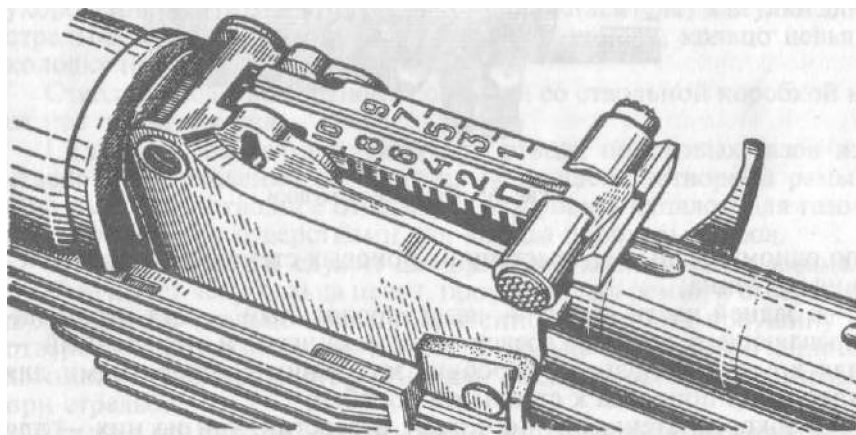
Рис. 57. Прицел
