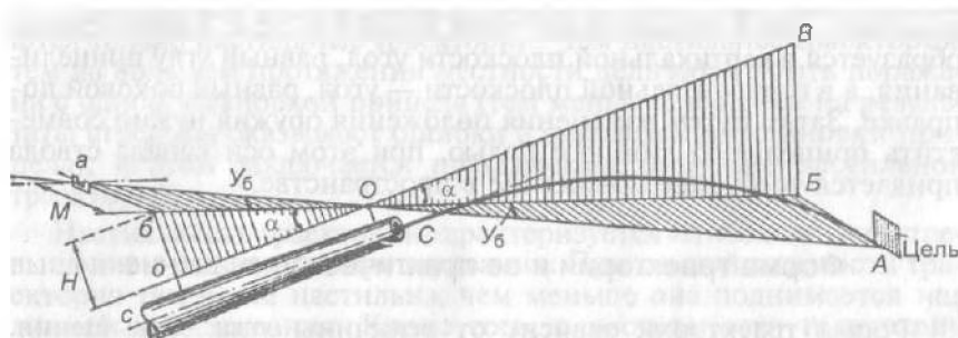
Рис. 13. Прицеливание (навodka) с помощью открытого прицела: O — мушка; a — целик; aO — прицельная линия; cC — ось канала ствола; oO — линия, параллельная оси канала ствола; Я — высота целика; M — величина перемещения целика; \alpha — угол прицеливания; Y_B — угол боковой поправки
