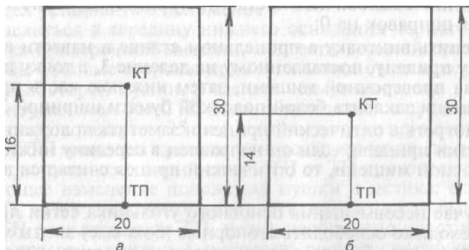
Рис. 148. Проверочные мишени: а — для открытого прицела; б — для оптического прицела. Размеры указаны в сантиметрах
