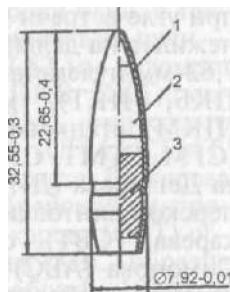
Рис. 140. 7,62-мм винтовочный снайперский патрон: а — патрон; б — пуля; 1 — оболочка; 2 — сердечник стальной; 3 — сердечник свинцовый
