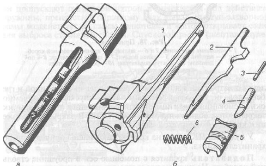
Рис. 77. Затвор:
