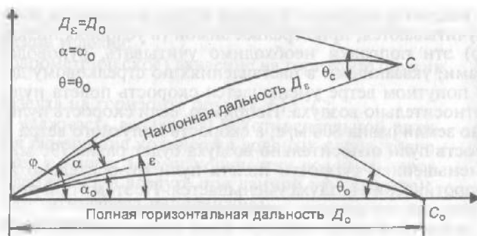
Рис. 20. Жесткость траектории
