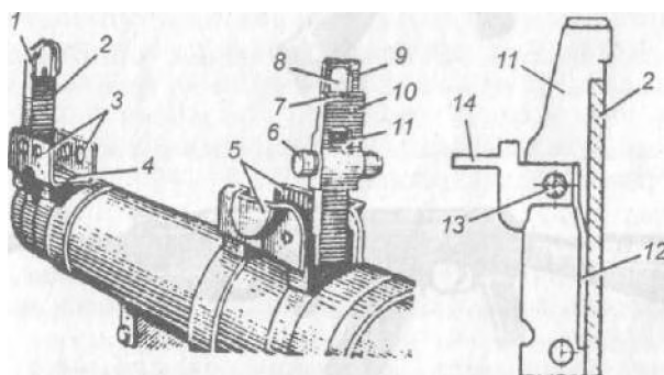
Рис. 94. Механический (открытый) прицел:
