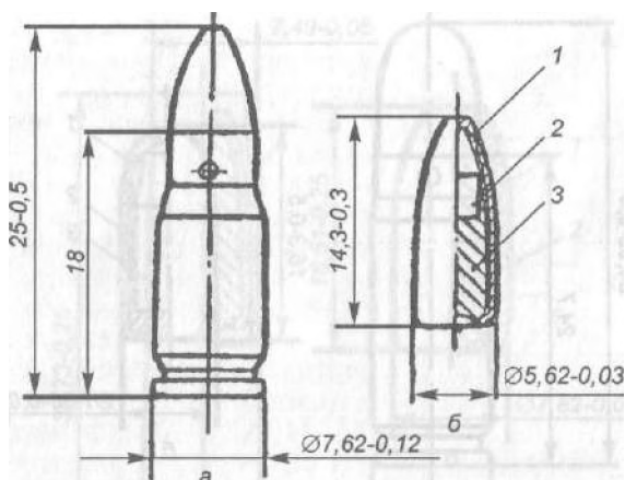
Рис. 127. 5,45-мм пистолетный патрон МПС: а — патрон; б — пуля; 1 — оболочка; 2 — сердечник стальной; 3 — сердечник свинцовый
