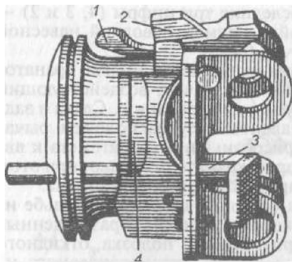
Рис. 100. Казенник:
